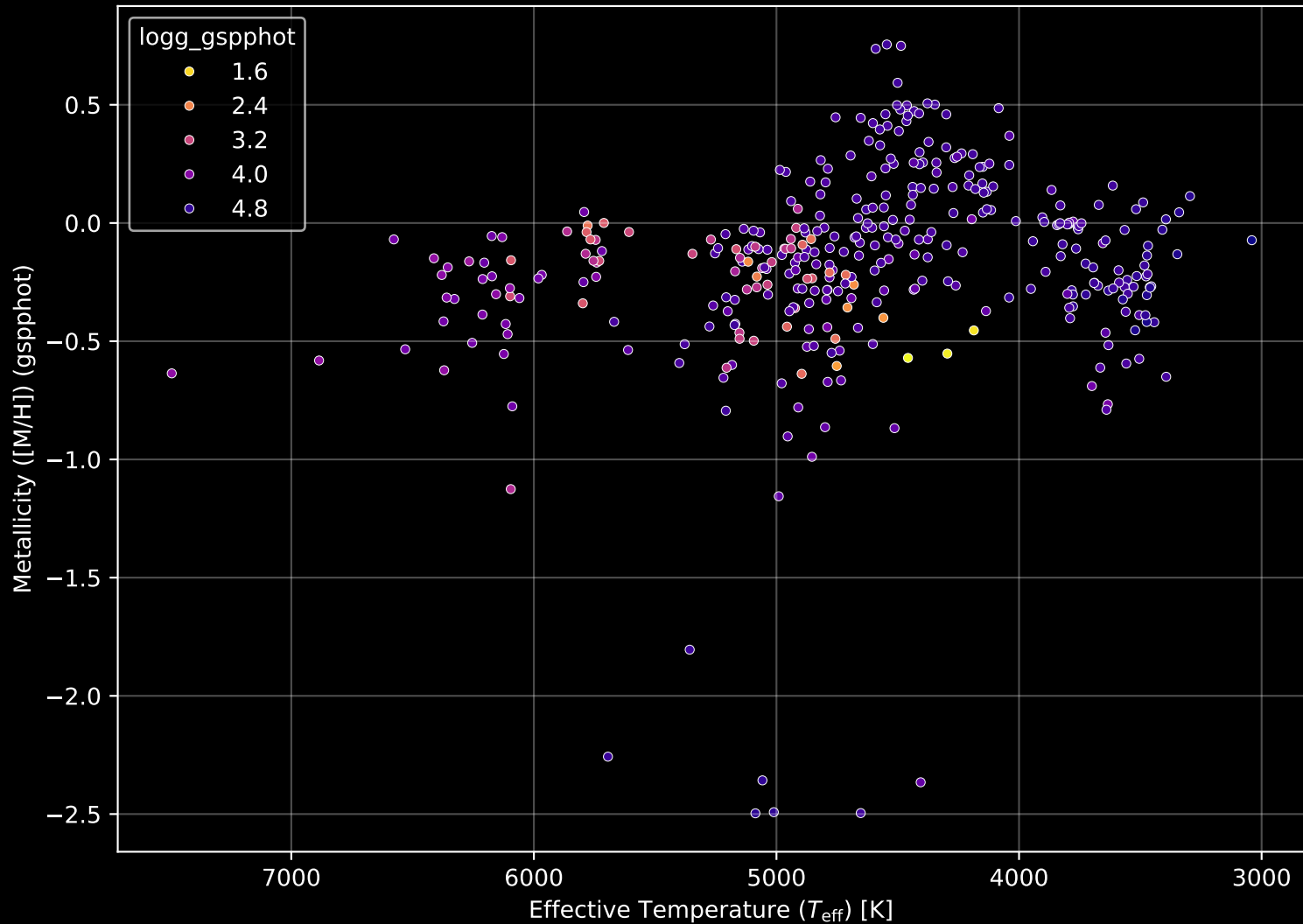
APOGEE DR17 Field: [090+75] Stellar Population Parameters (n= 366)
